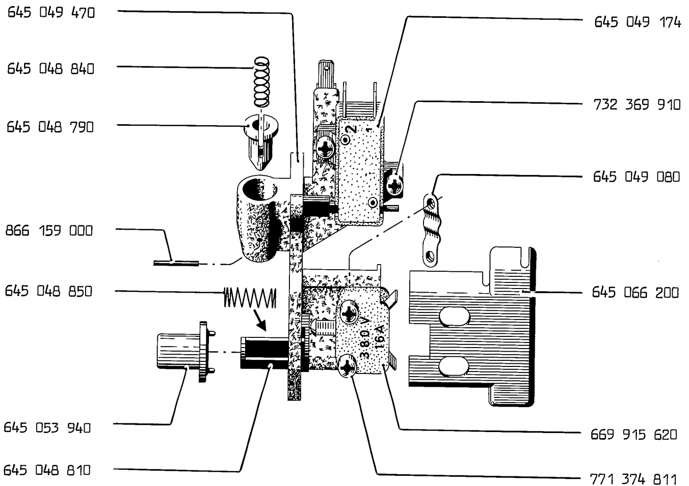
Elektrische Türverriegelung
